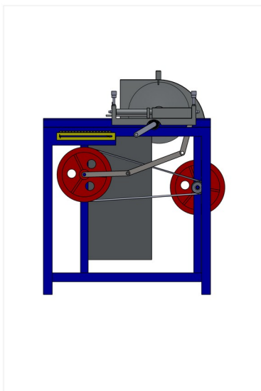
Tampak Belakang
