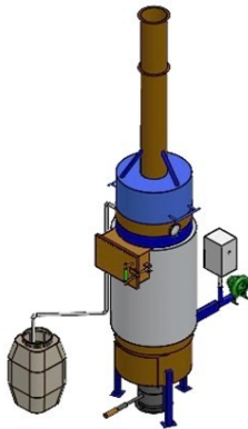
Gambar 7 Tampak Perspektif
