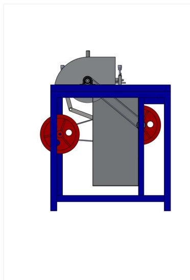
Tampak Depan
