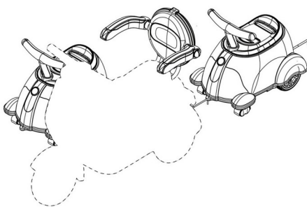
Gambar 5 : Perspektif Depan
