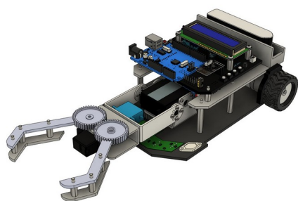
Tampak Perspektif
