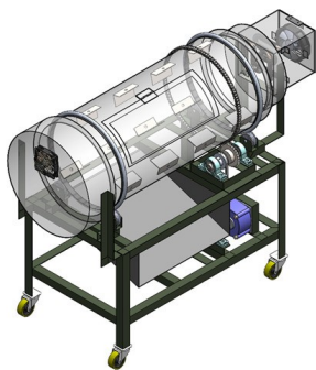
Tampak Perspektif
