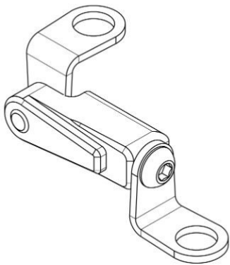
Tampak Perspektif
