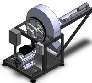
Tampak Perspektif
