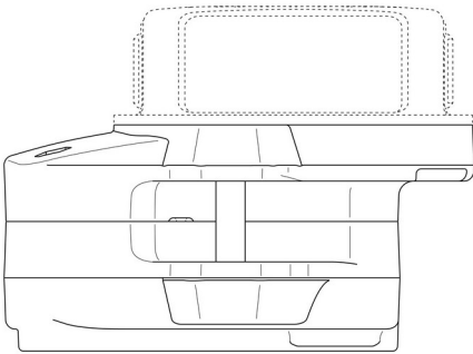
Tampak Atas
