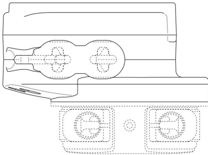
Tampak Bawah
