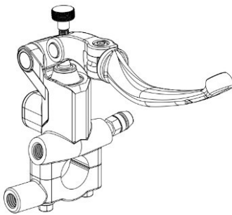
Tampak Perspektif
