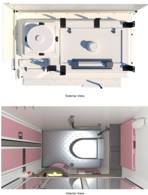
Tampak Atas
