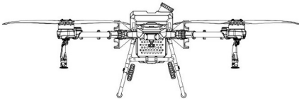
Tampak Belakang
