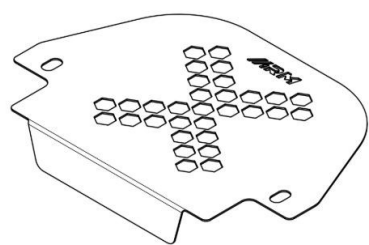
Tampak Perspektif
