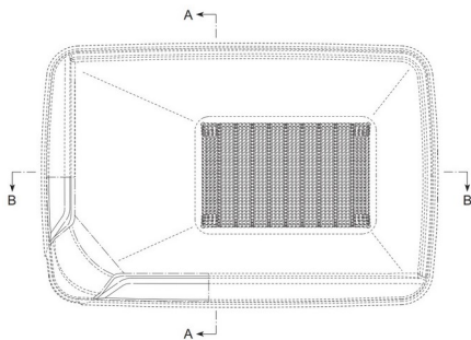
Tampak Atas
