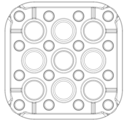
Tampak Bawah
