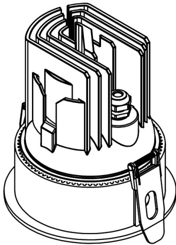
Tampak Perspektif
