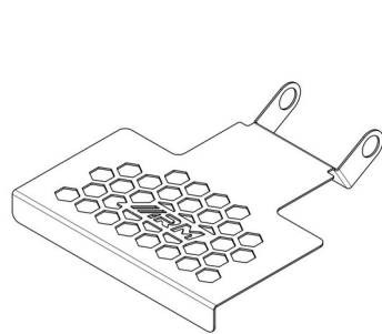
Tampak Perspektif
