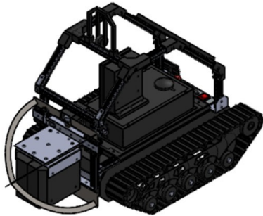
Tampak Perspektif
