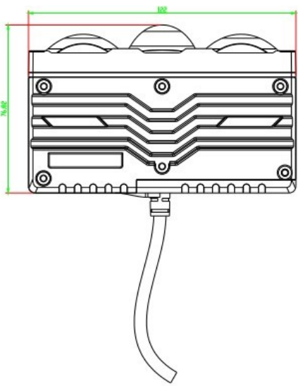
Tampak Bawah
