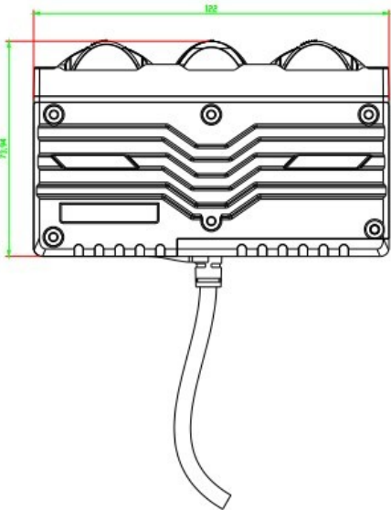
Tampak Bawah
