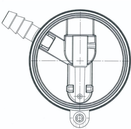
Tampak Atas
