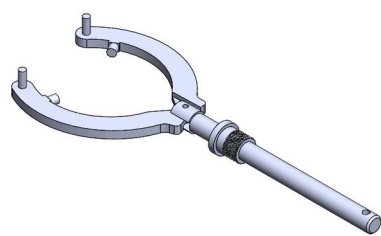
Tampak Perspektif
