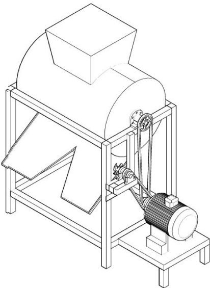
Tampak Perspektif
