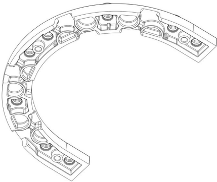
Tampak Perspektif
