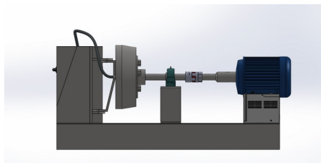
Tampak Depan
