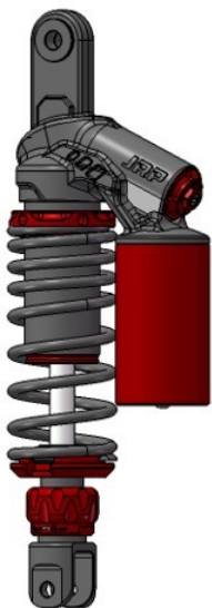
Tampak Perspektif
