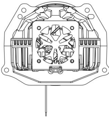
Tampak Belakang
