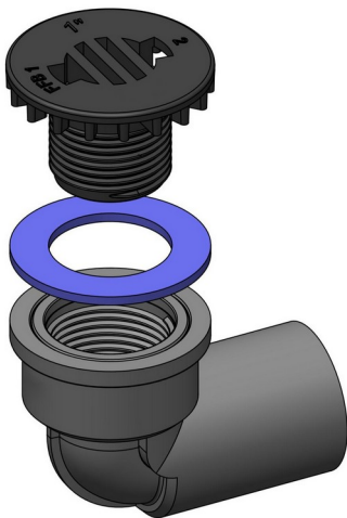
Tampak Perspektif
