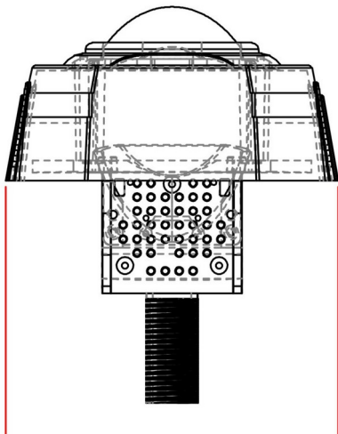
Tampak Bawah
