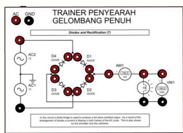
Tampak Atas
