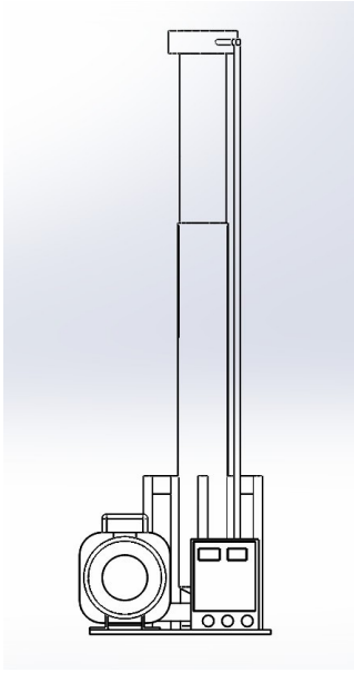
Tampak Belakang
