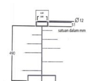
Gambar Desain
